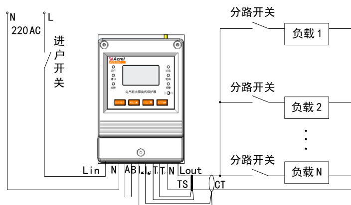
ASCP200-1 型限流式保护器的应用接线图
