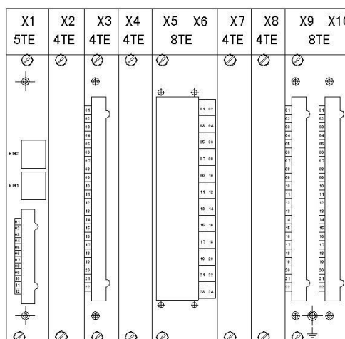
ARB5-M(ARB5-E)后面板
