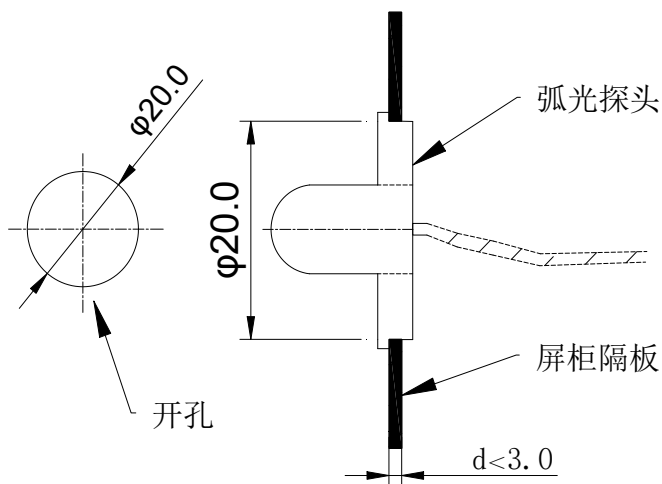
ARB5-S 弧光探头开孔尺寸及安装示意图
